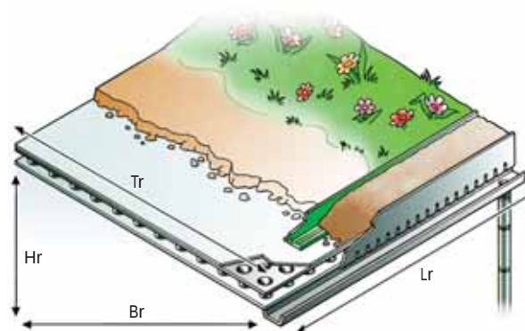
Bild 1. Dachabmessung
