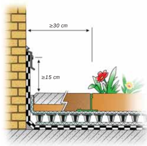
Detail 2. Fassade
