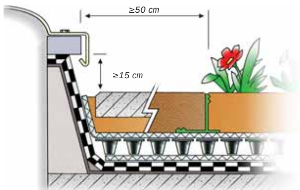
Detail 5. Lichtkuppel
