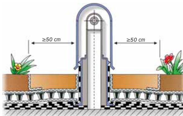
Detail 6. Fallschutz / Sekurant
