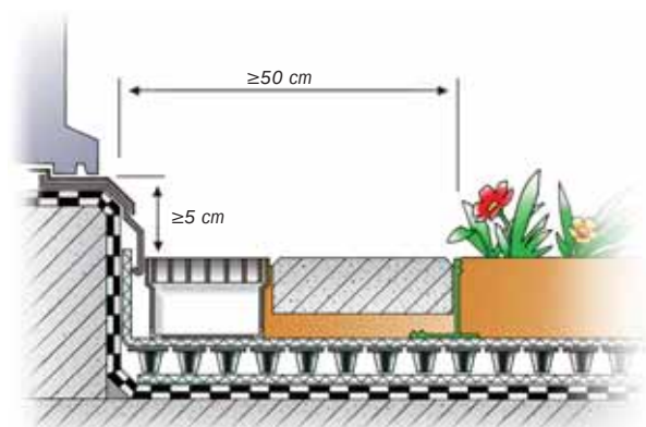
Detail 1. Türaustritt
