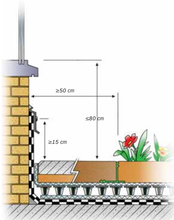
Detail 3. Fassade mit z.B. Fensteröffnung ≤ 80 cm über Oberkante Substrat
